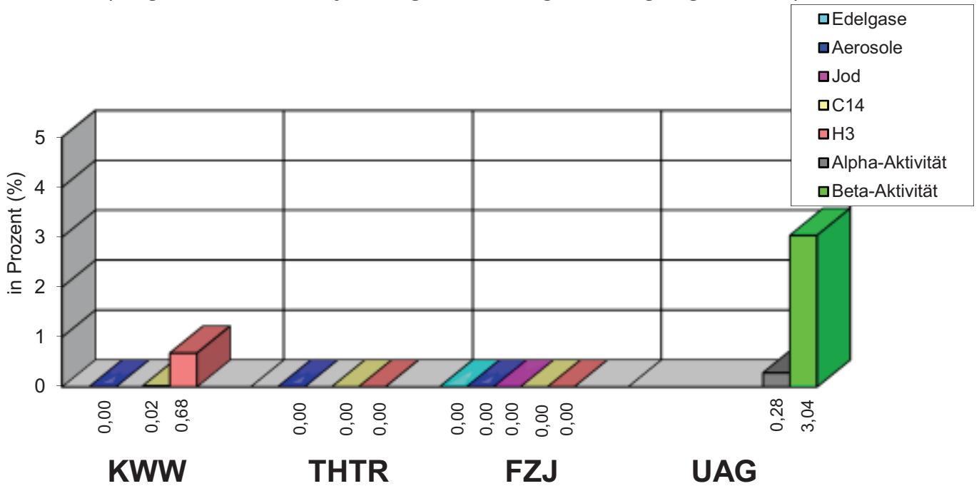
Aktivitätsabgaben mit der Luft (Angaben in % des jeweiligen Jahresgenehmigungswertes)
